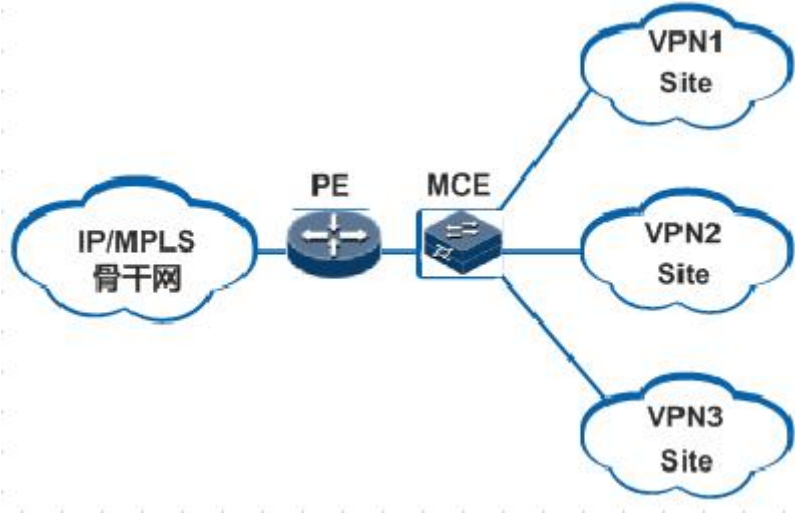
图 11-2 部署 MCE 后的组网
