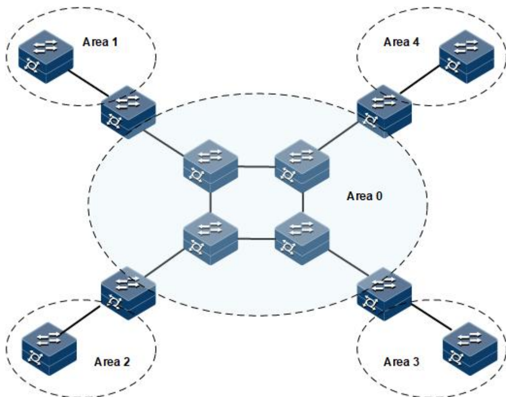
图 3-20 OSPF 区域划分
