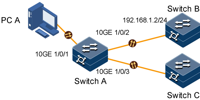
图 3-5 配置策略路由组网示意图
