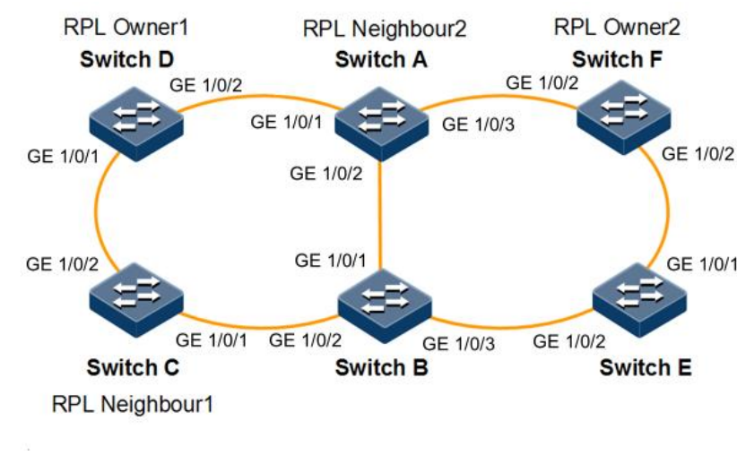
图 9-8 相交环 G.8032 应用组网示意图
