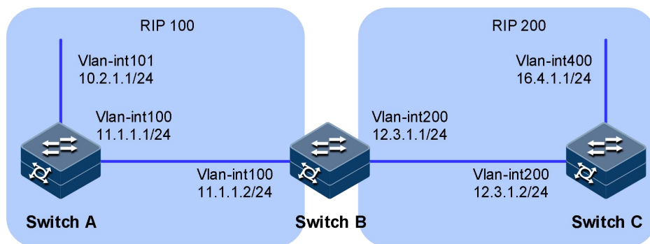
图 3-48 RIP 引入外部路由配置组网图
