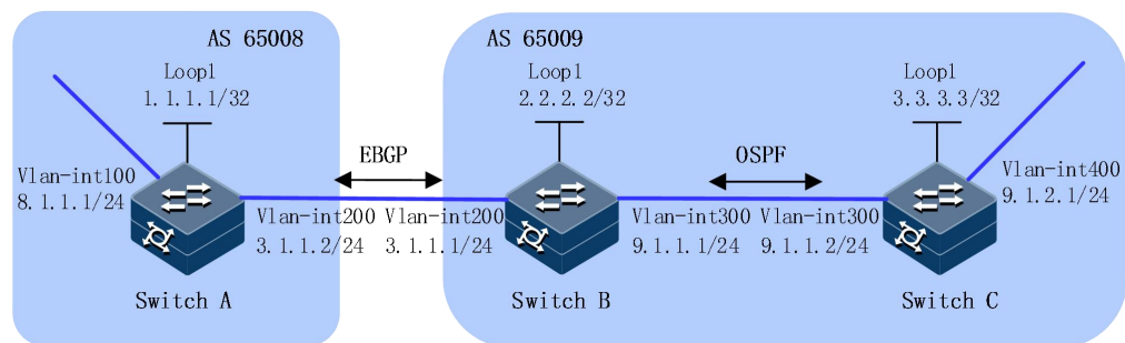
图 3-14 BGP 与 IGP 交互配置组网图
