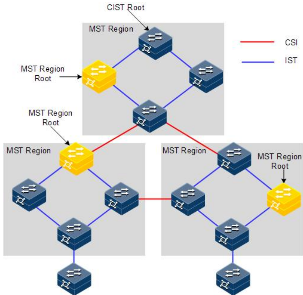
图 9-13 MSTP 网络基本概念示意图
