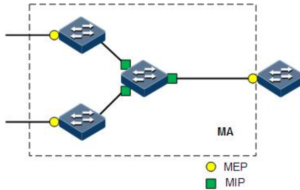
图 7-7 不同级别 MD 网络示意图
