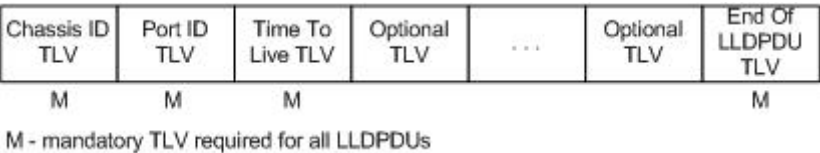
图 10-7 LLDPDU 结构图
