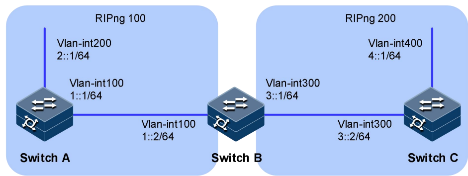
图 3-50 RIPng 引入外部路由组网图
