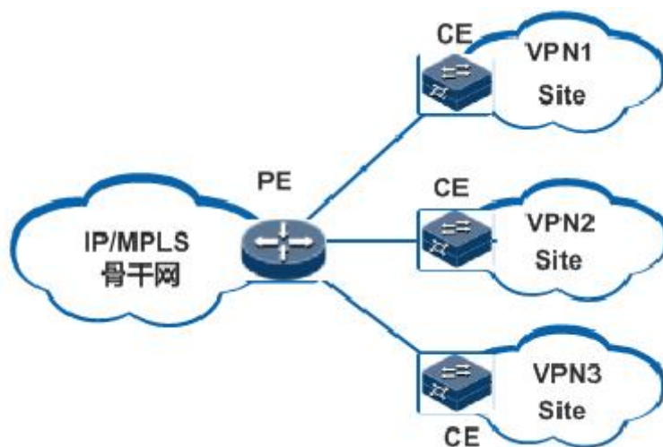
图 11-1 部署 MCE 前的组网
