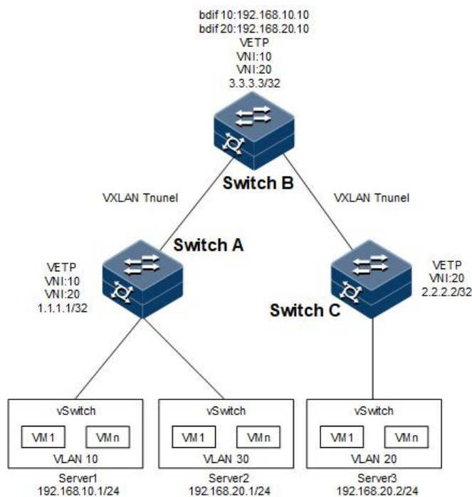
图 12-4 BGP EVPN 方式集中式网关组网图
