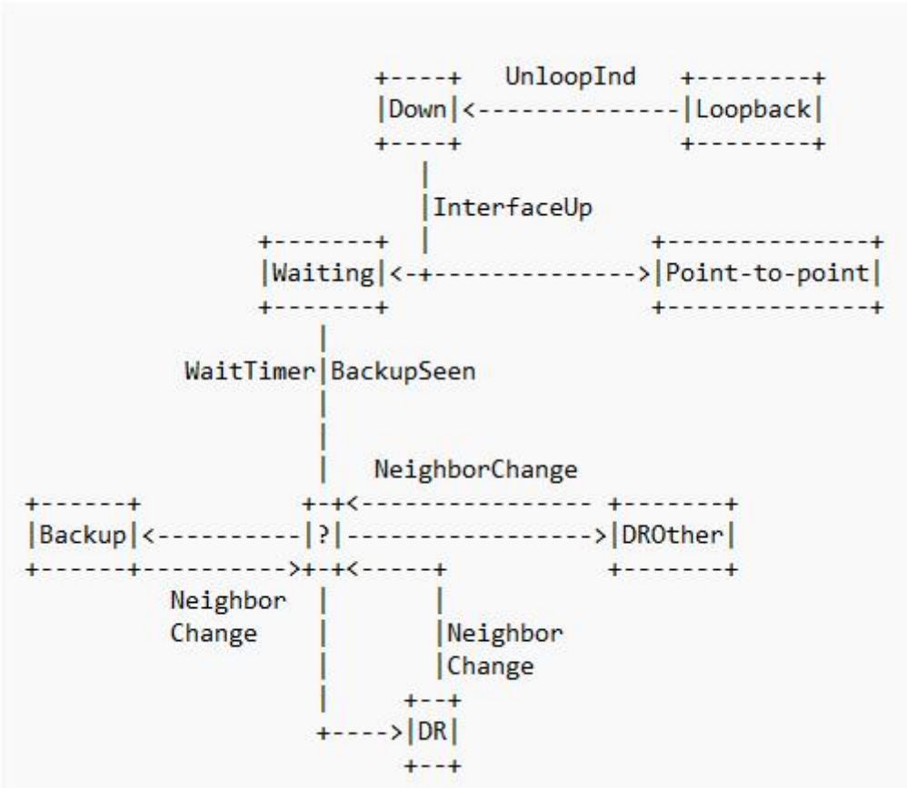
图 3-23 OSPF 接口状态机
