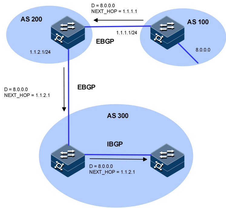
图 3-7 NEXT_HOP 属性
