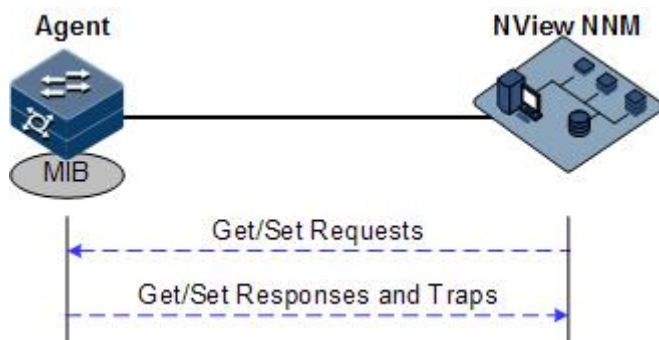
图 10-1 SNMP 工作机制示意图
