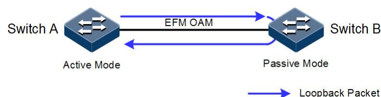
图 7-1 OAM 环回示意图
