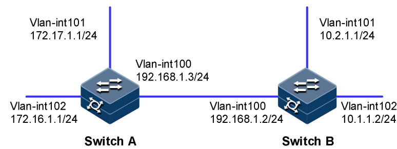
图 3-47 RIP 基本功能组网图
