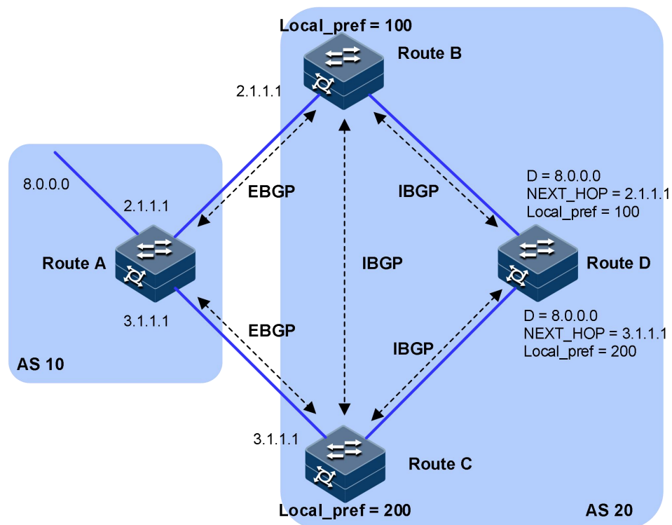
图 3-9 LOCAL_PREF 属性
