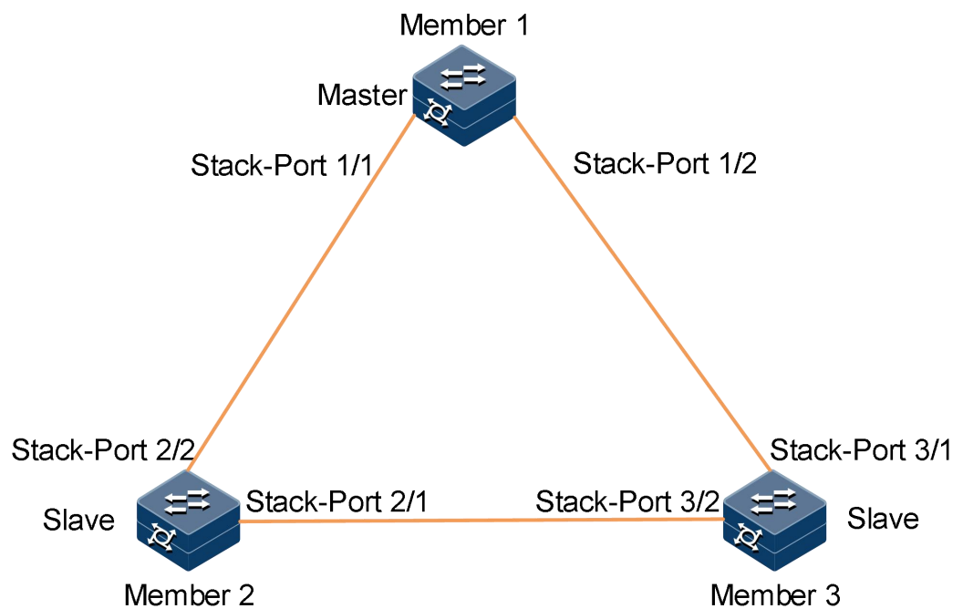
图 10-17 3 台成员设备组成环形型拓扑
