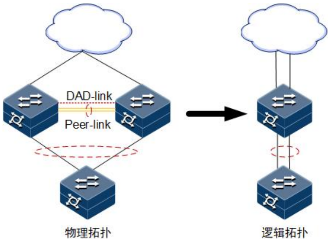
图 2-14 M-LAG 物理拓扑视图与逻辑拓扑视图
