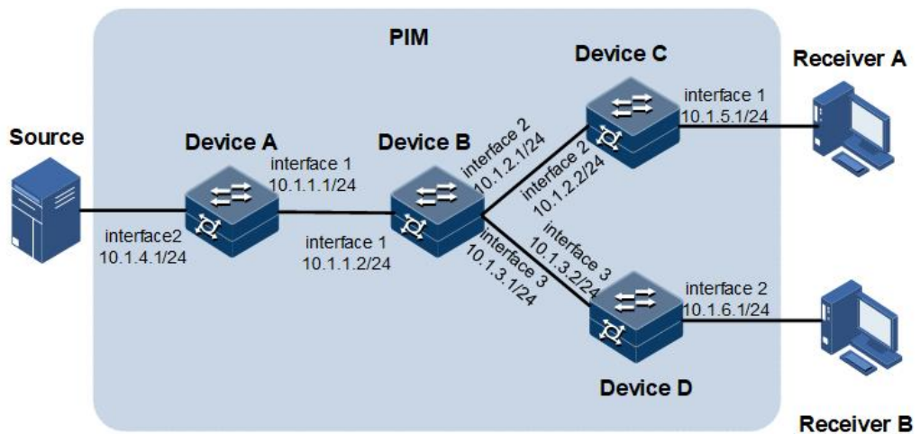
图 6-20 PIM-DM 功能功能组网应用示意图
