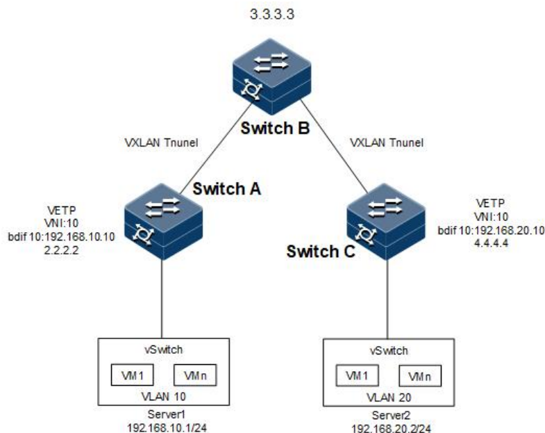
图 12-5 BGP EVPN 方式分布式网关组网图
