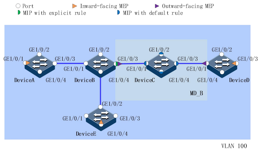
图 7-8 CFM 典型配置组网图
