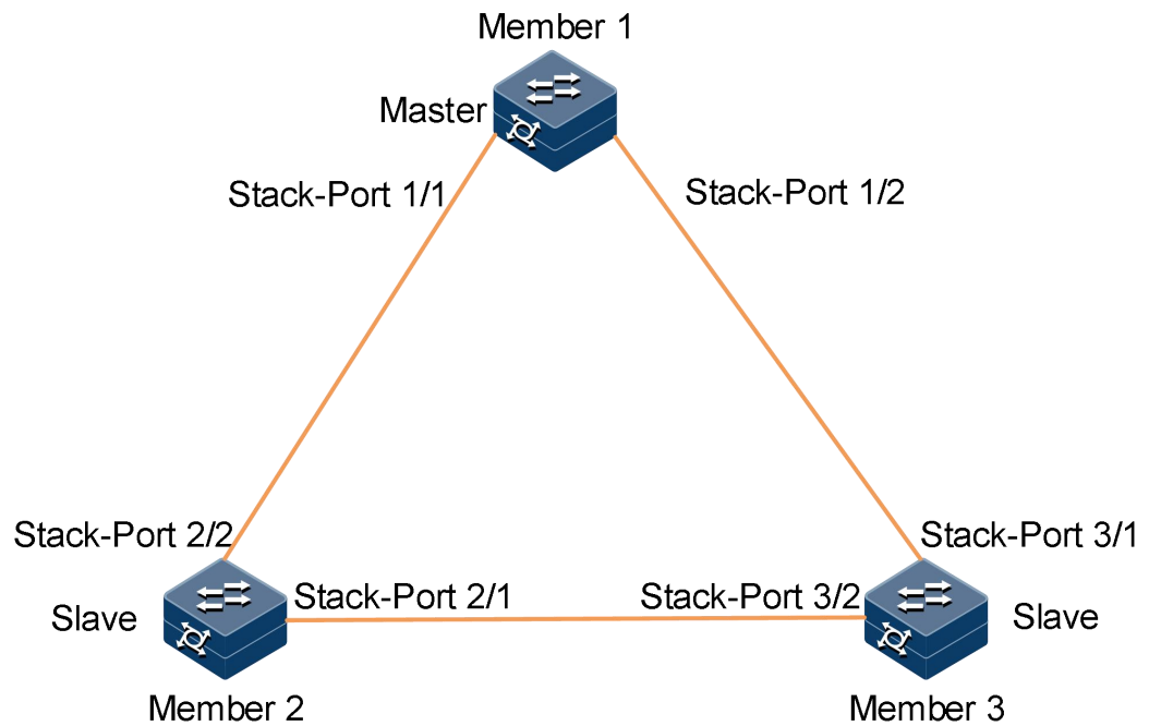
图 10-18 3 台堆叠拓扑图
