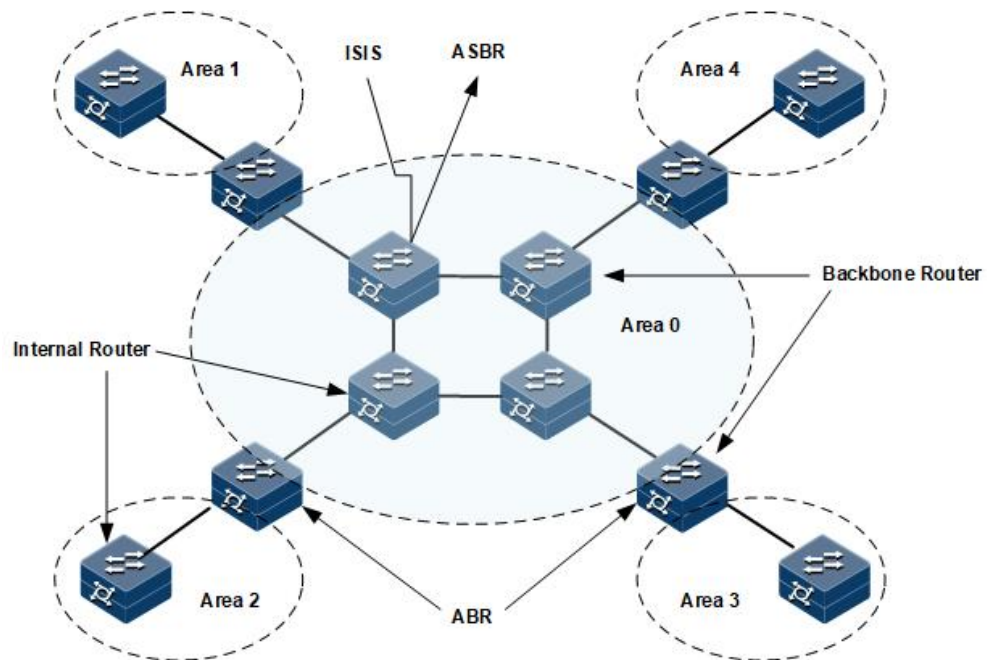
图 3-21 OSPF 路由器类型示例
