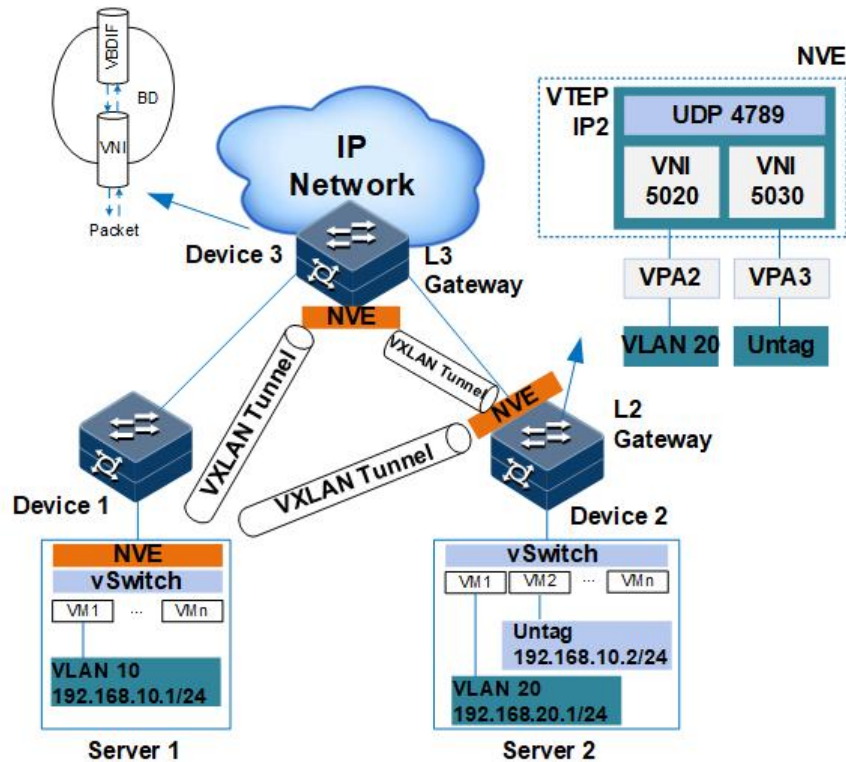
图 12-1 VXLAN 结构示意图
