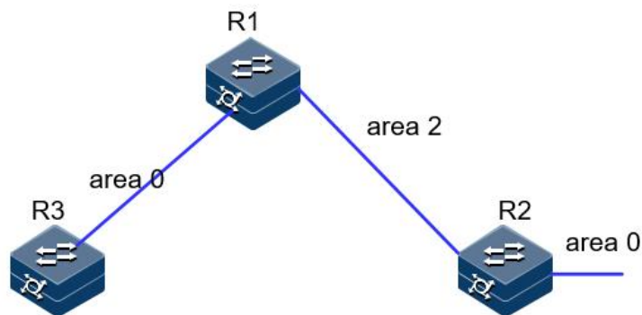
图 3-31 配置 OSPF 虚连接的组网图
