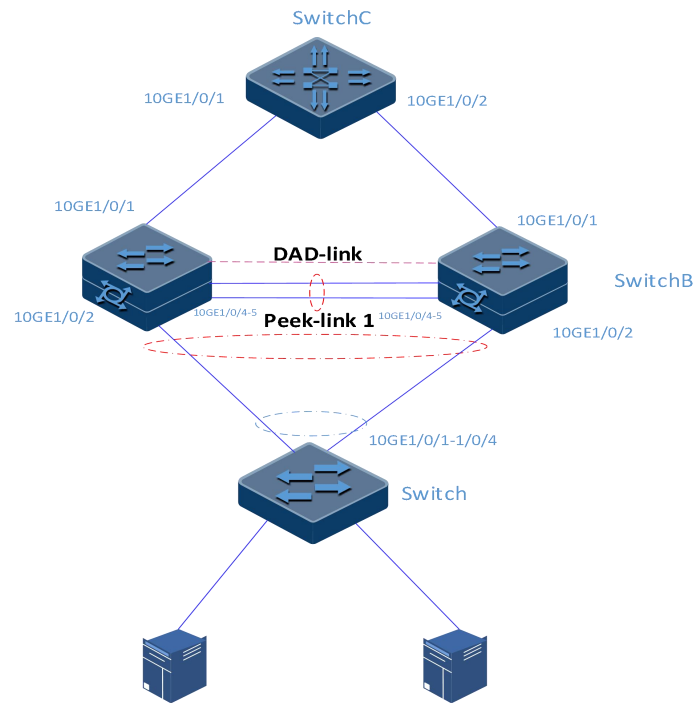
图 2-15 配置 M-LAG 双归接入 IP 组网图
