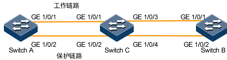
图 9-2 G.8031 组网示意图
