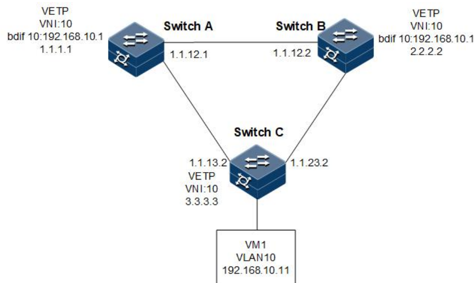
图 12-6 多活网关组网图
