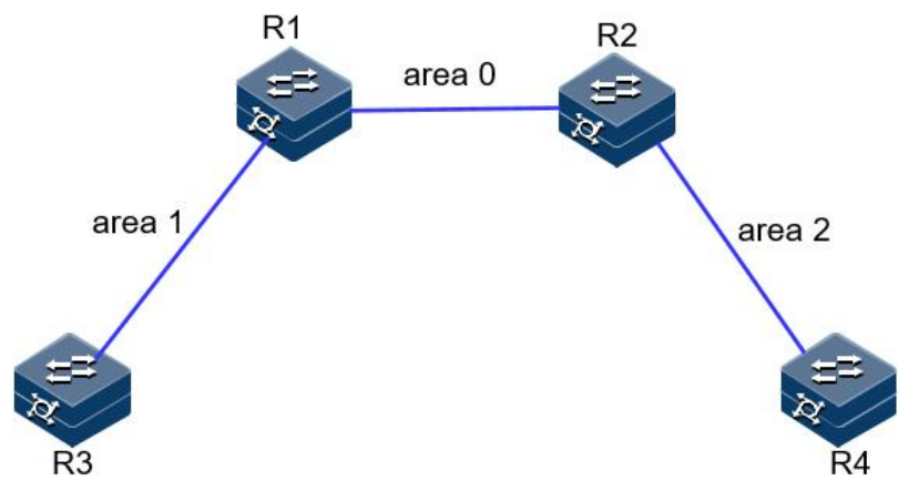
图 3-39 OSPFV3 基本配置组网图
