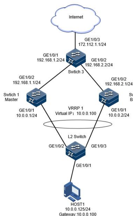
图 7-5 配置 VRRP 主备组网图
