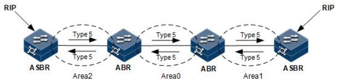
图 3-25 OSPFNSSA 区域示意图
