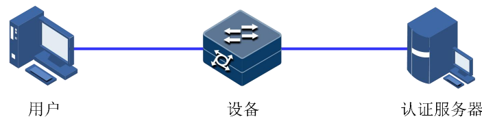
图 8-15 MAC 认证组网示意图
