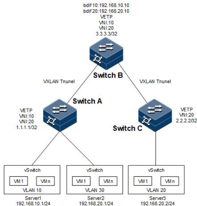
图 12-3 静态方式集中式组网图
