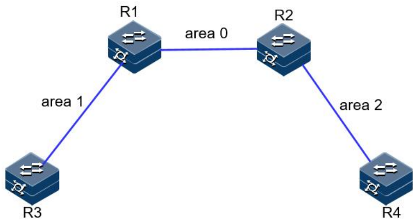
图 3-27 OSPF STUB 区域示例组网图
