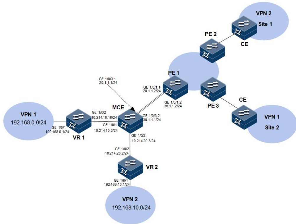
图 11-3 MCE 典型配置示意图
