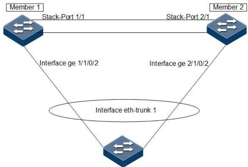
图 10-20 MAD 代理模式
