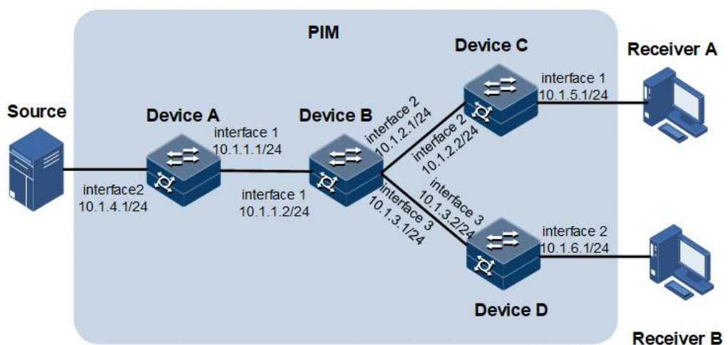
图 6-21 PIM-SM 功能功能组网应用示意图
