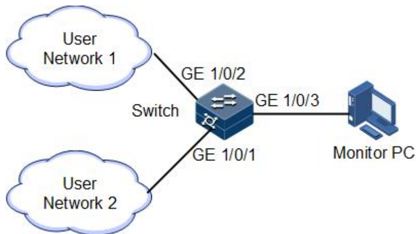
图 10-11 接口镜像应用组网示意图
